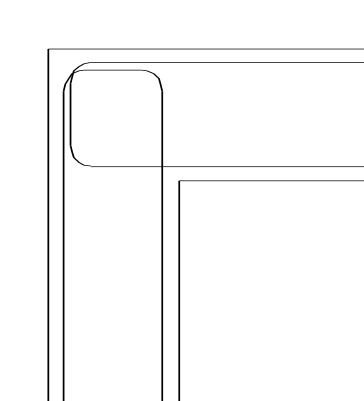
Figur 6:42a. Armeringsutförande vid anslutning inom hörnområde mellan konstruktionsdelar i skyddsrummets stomme
