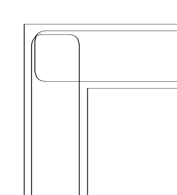
Figur 6:42a. Armeringsutformning vid anslutning inom hörnområde mellan konstruktionsdelar i skyddsrummets stomme
