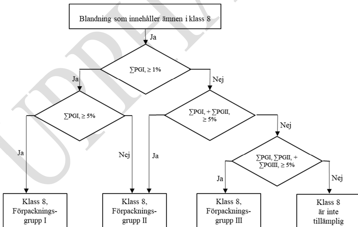
Figur 2.2.8.1.6.3: Beräkningsmetod
